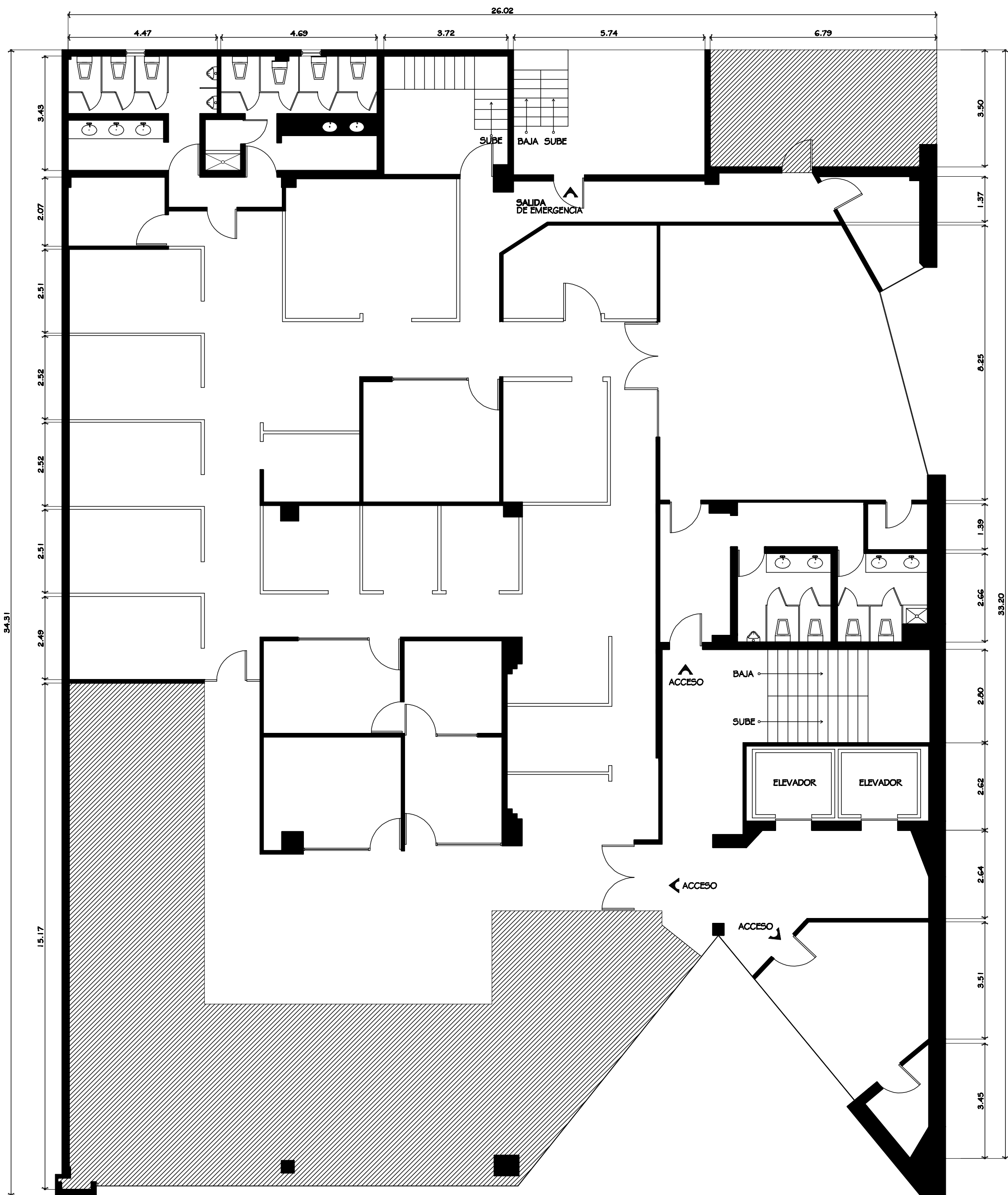
PLANTA PISO 8 ESC. 1:100
