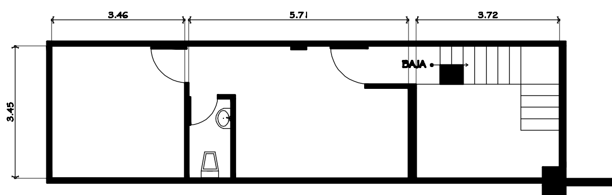
PLANTA ALTA PISO 8 ESC. 1:100
